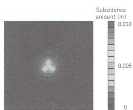
(d) Filler 3 ( q_u=1.0 )
