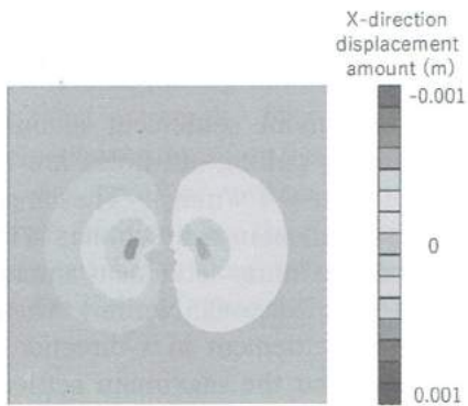
(d) Filler 3 ( q_u=1.0 )
