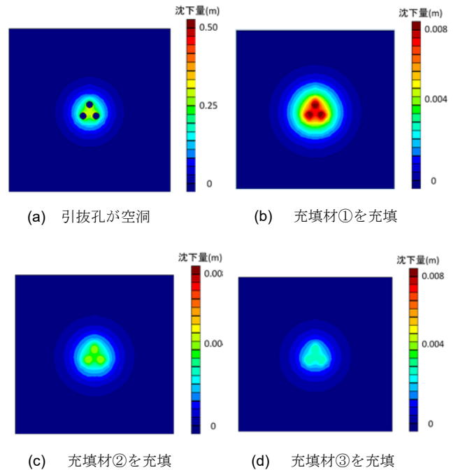
図-2 地表面における沈下量コンター図
