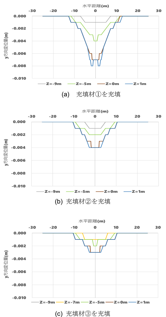
図-3 充填時におけるy方向変位量
