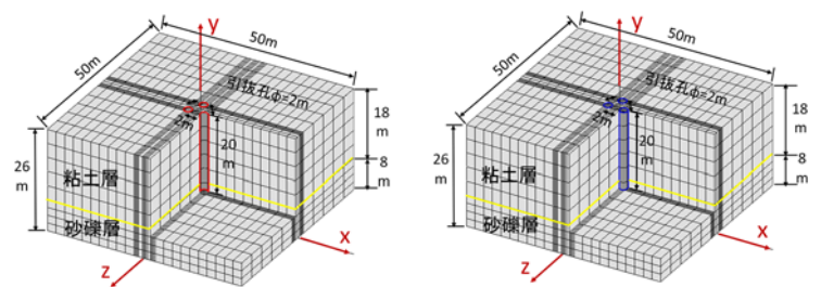
(a) 引抜孔が空洞の場合 (b) 引抜孔を充填した場合
